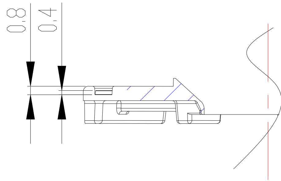
C-C
